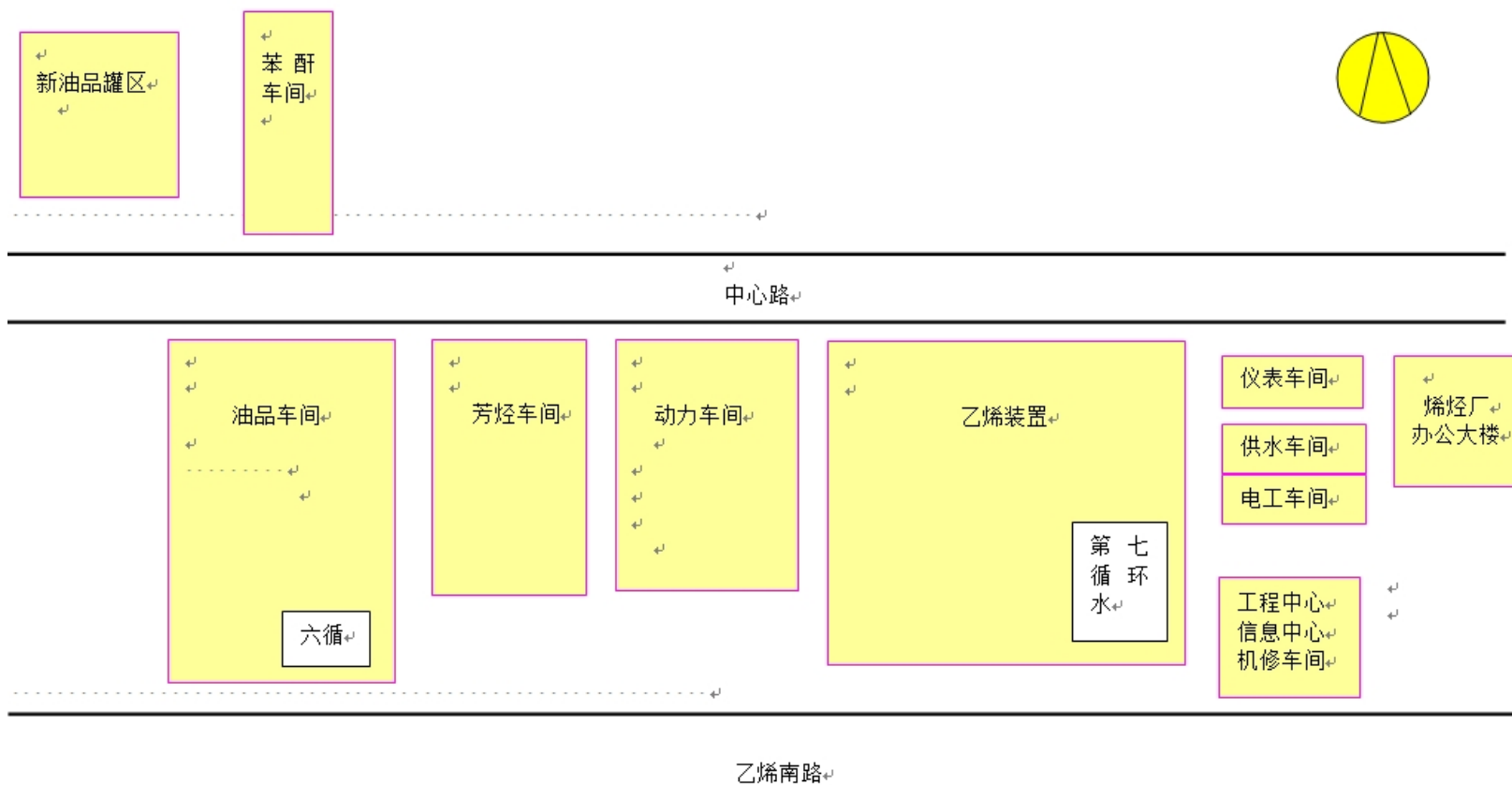
图 3-1 烯烃厂平面布置图
