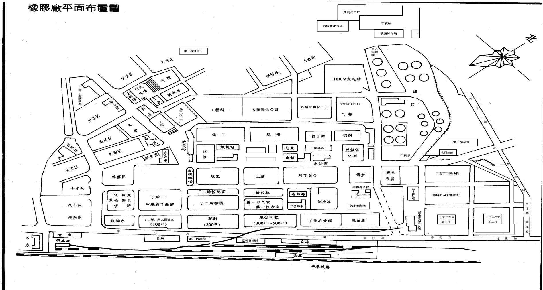
图 3-1 橡胶厂平面布置图
