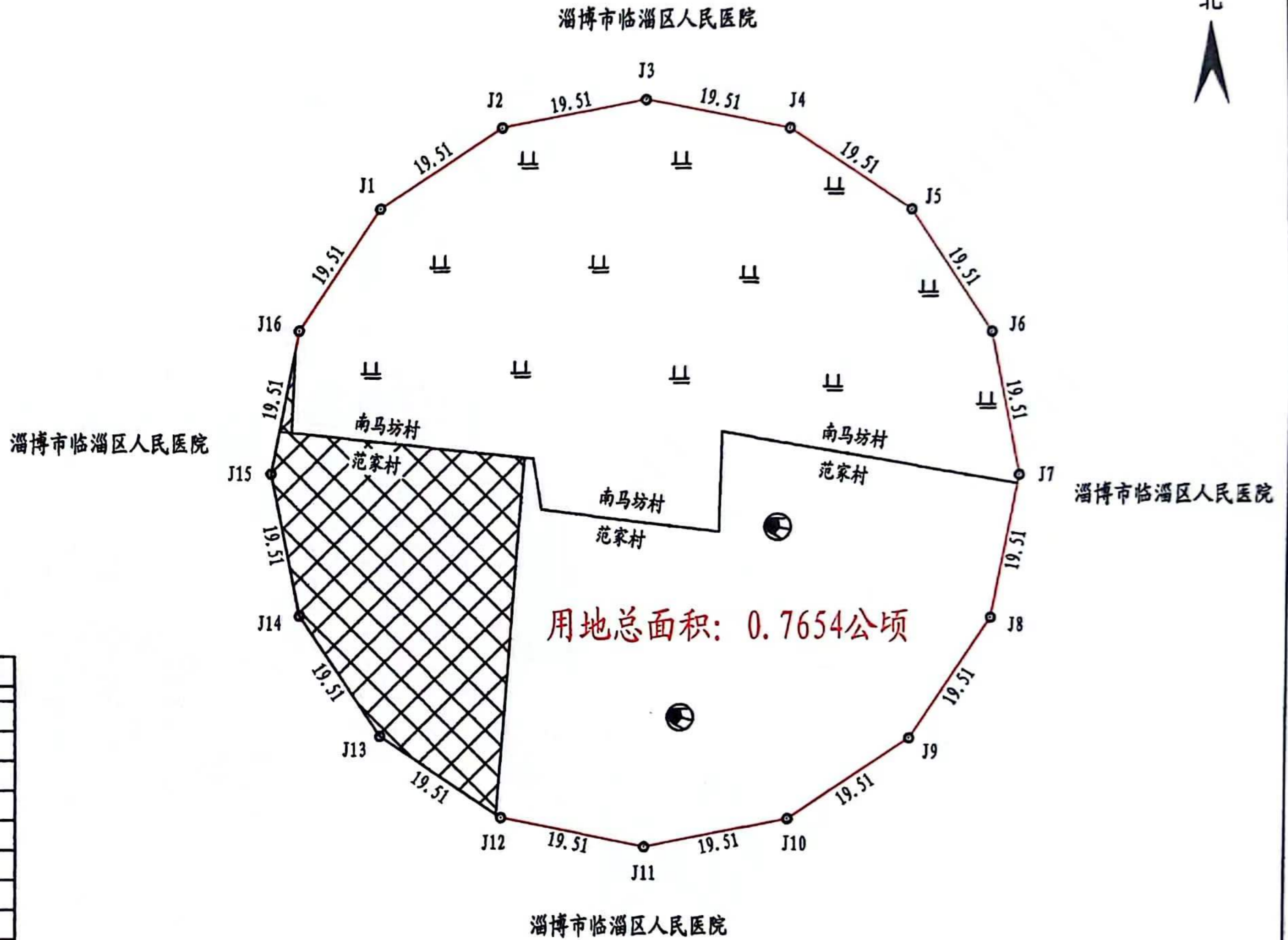
界址点坐标表 2000国家大地坐标系117度
