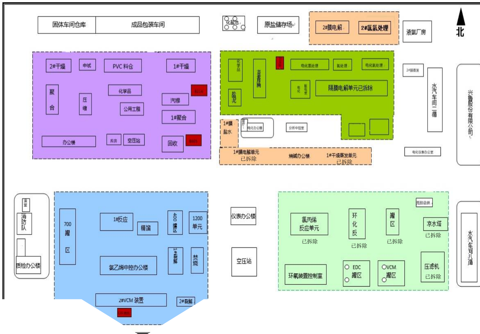
图 3-1 氯碱厂平面布置图
